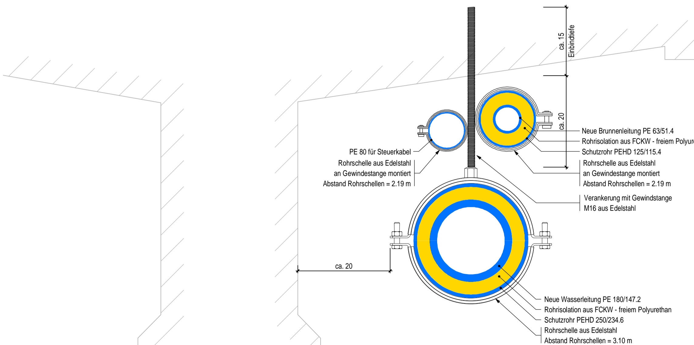
Detail Rohraufhängung Sisslenbrücke 1:5
