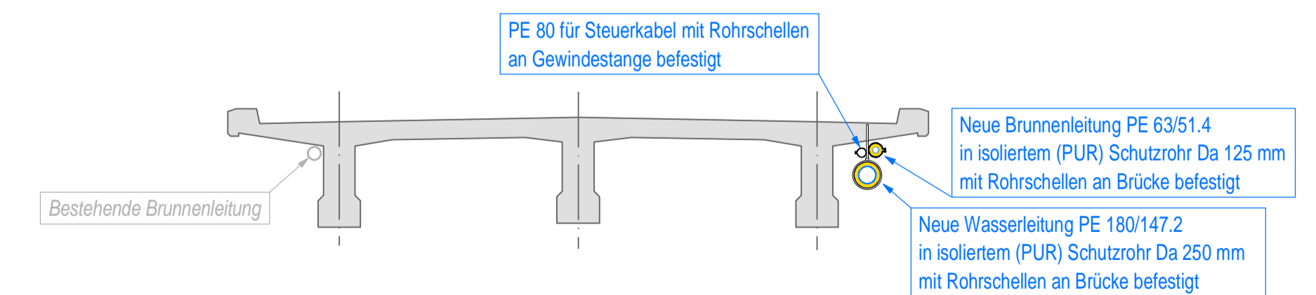
Schnitt A - A Sisslenbrücke 1:50
